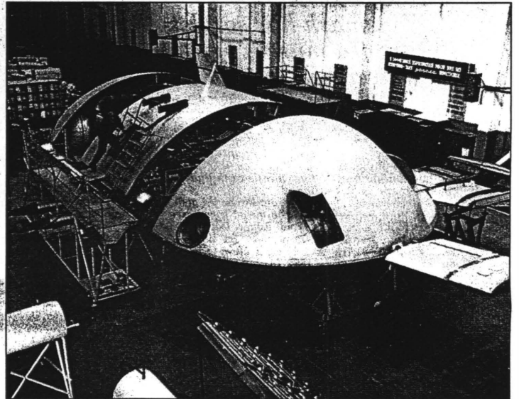
En ni ton tung fuldskalamodel af EKIP på flyvebasen i Saratov.
