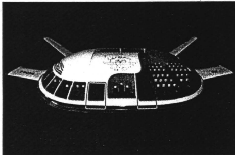
Model af passagerudgaven af EKIP. Den vejer 35 ton, har plads til 80 passagerer og når en maksimumhastighed af 650 km/t. Den kan nøjes med en startbane på 450 meter.
